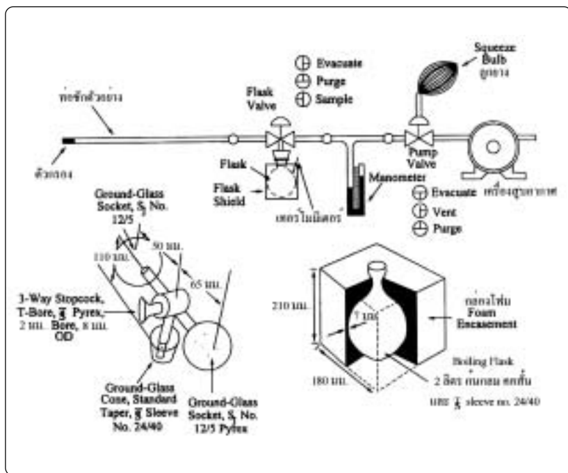
ภาพที่ 7-1 แสดงชุดเก็บตัวอย่าง วาล์วขวดเก็บตัวอย่าง และขวดเก็บตัวอย่าง
