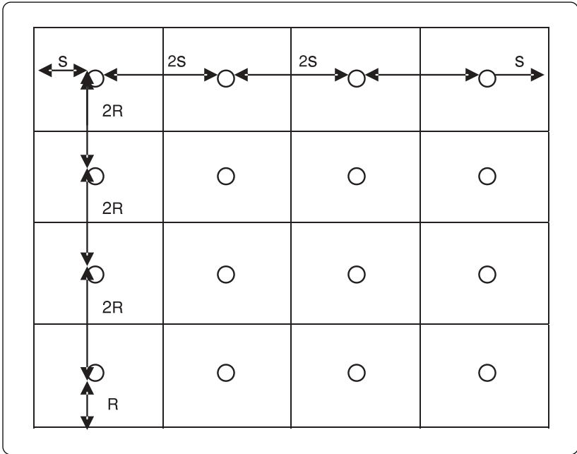
ภาพที่ 1-7 แสดงการกำหนดตำแหน่งจุดชักตัวอย่าง 16 จุด ของปล่องที่มีลักษณะทรงสี่เหลี่ยม
