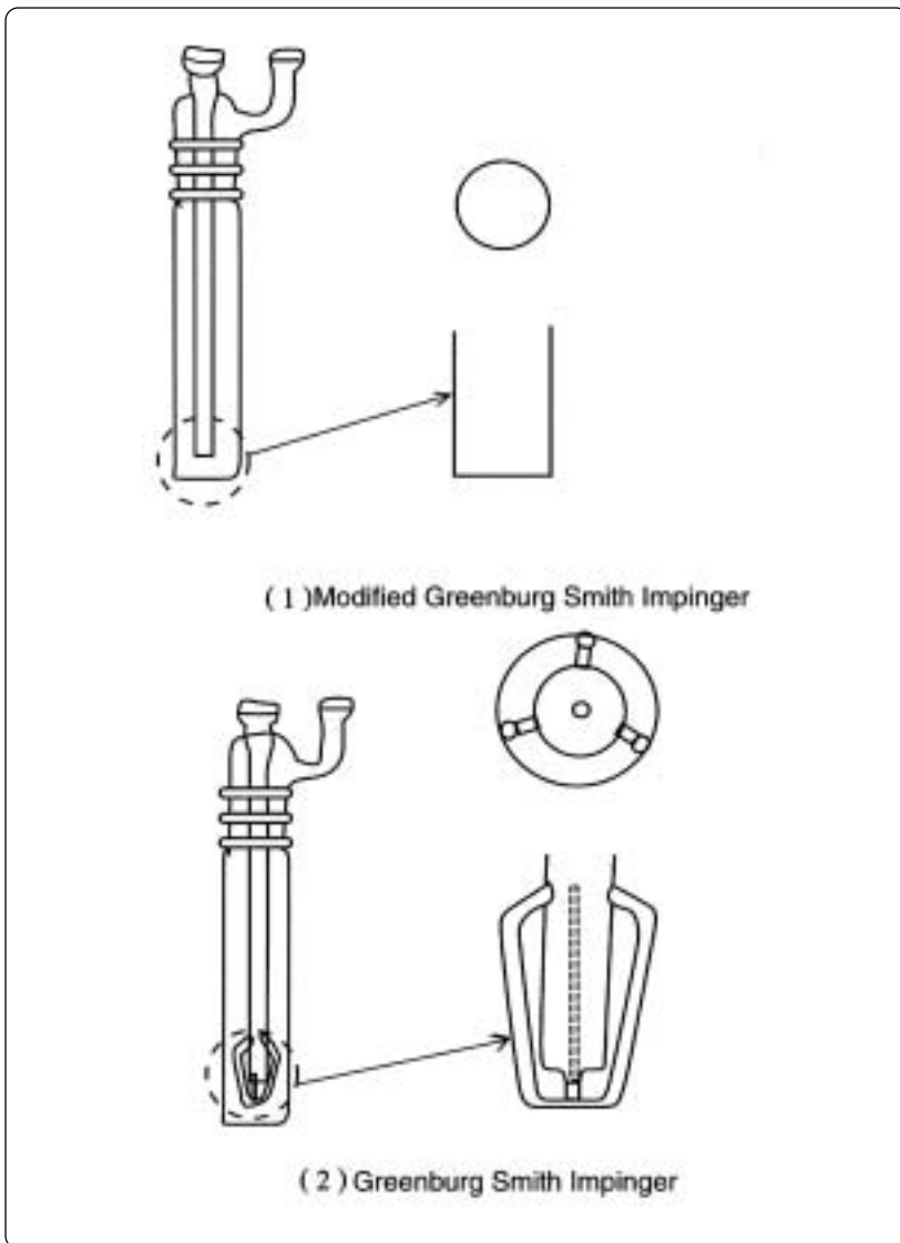
ภาพที่ 5-4 แสดงลักษณะของ Impinger
