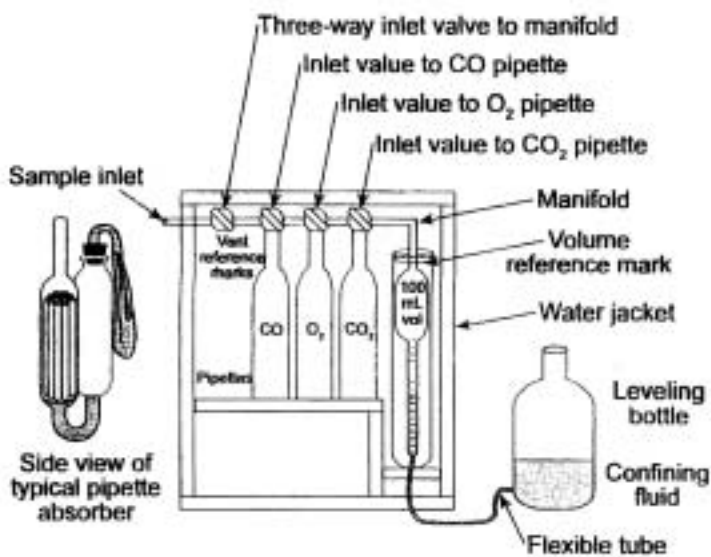
ภาพที่ 3-3 ชุดวิเคราะห์ Orsat สำหรับตรวจวัด \%O_2 , \%CO_2 และ \%CO
