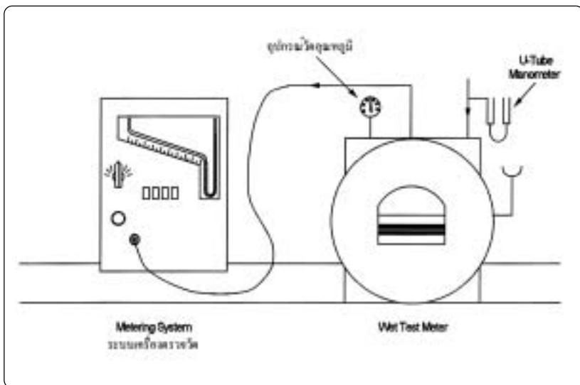
ภาพที่ 5-8 แสดงการจัดเรียงอุปกรณ์ในการปรับเทียบความถูกต้องของระบบเครื่องตรวจวัด
