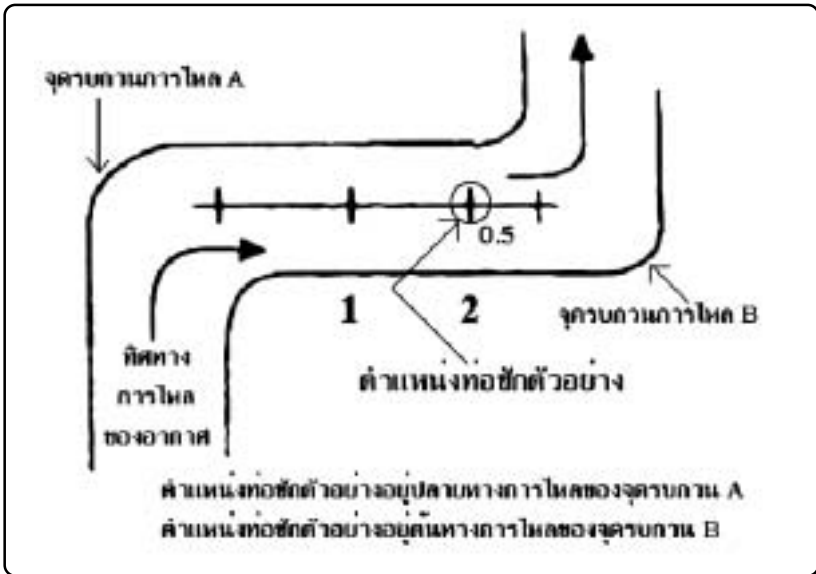
ภาพที่ 1-2 จุดเจาะปล่องที่ไม่เหมาะสม
