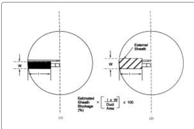
ภาพที่ 2-7 แสดงลักษณะการวาง Type S Pitot Tube ภายในปล่อง
