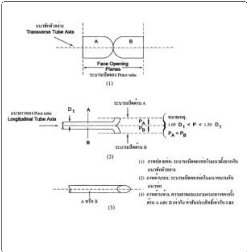
ภาพที่ 2-2 แสดงลักษณะที่ถูกต้องของ Type S Pitot Tube
