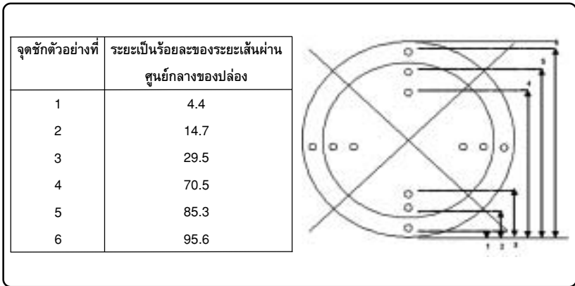
ภาพที่ 1-6 แสดงตัวอย่างการวางตำแหน่งจุดชักตัวอย่างบนพื้นที่ภาคตัดขวางของปล่องที่แบ่งเป็นพื้นที่
