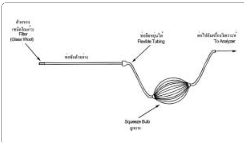
ภาพที่ 3-1 ชุดชักตัวอย่างอากาศแบบแยก (Grab Sampling Train)
