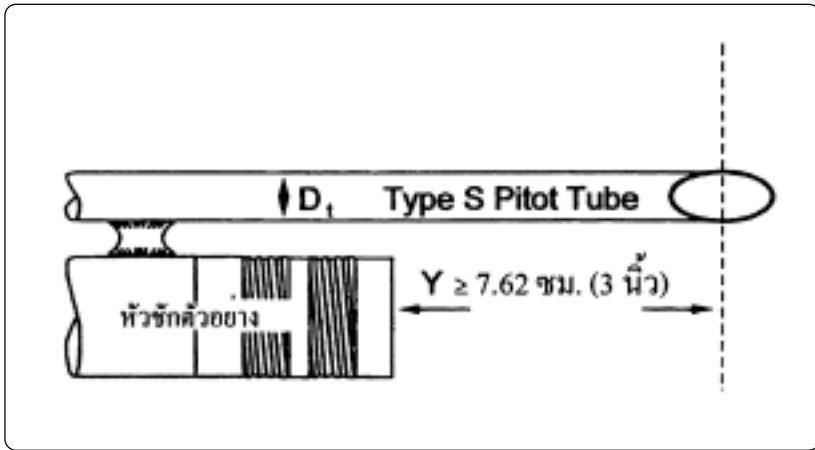
ภาพที่ 2-6 แสดงระยะห่างอย่างต่ำระหว่าง Type S Pitot Tube กับหัวชักรั่วอย่างเพื่อป้องกันสิ่งรบกวน
