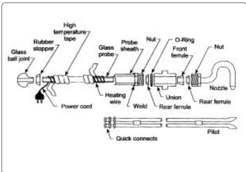
ภาพที่ 5-1ก แสดงรายละเอียดของท่อชักตัวอย่าง
