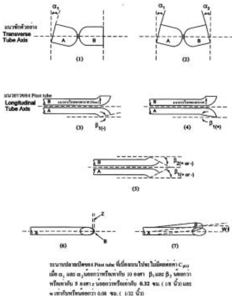
ภาพที่ 2-3 แสดงระนาบปลายเปิดของ Type S Pitot Tube ซึ่งมีการเบี่ยงเบนไป
