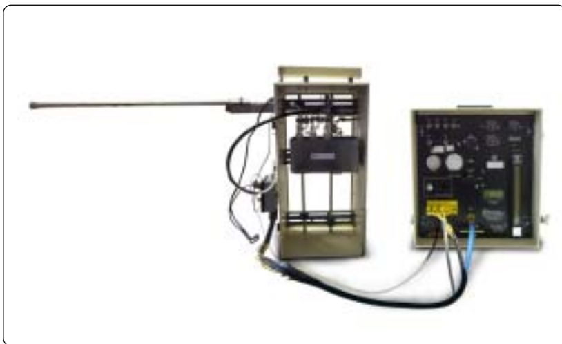
ภาพที่ 6-2 แสดงชุดเก็บตัวอย่างซัลเฟอร์ไดออกไซด์
