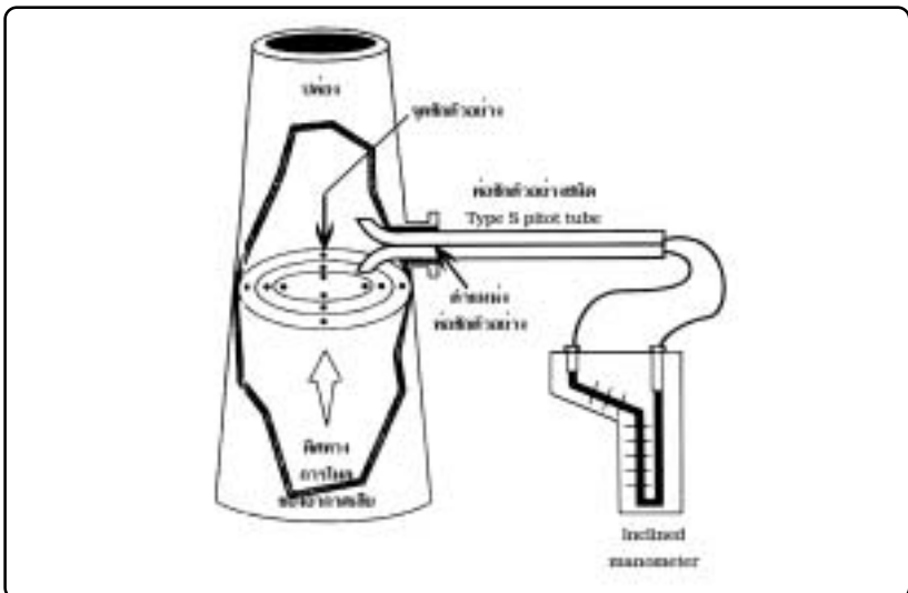
ภาพที่ 1-1 จุดเจาะปล่อง และจุดชักตัวอย่าง
