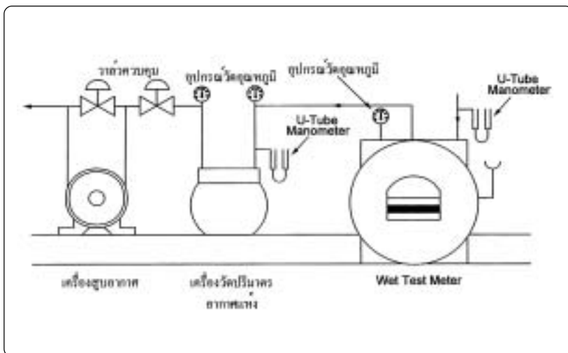
ภาพที่ 5-9 แสดงการจัดเรียงอุปกรณ์ในการปรับเทียบความถูกต้อง เครื่องวัดปริมาตรอากาศแห้ง
