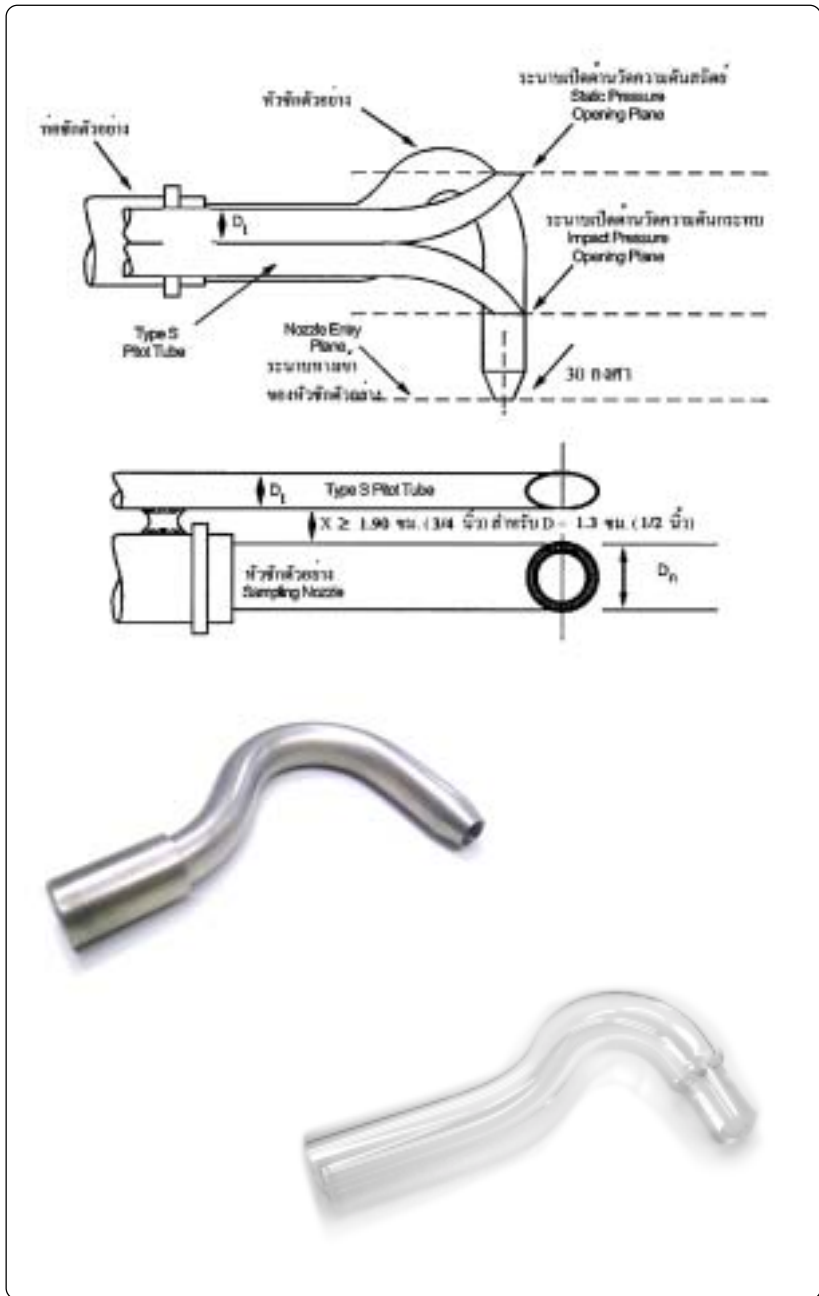
ภาพที่ 5-2 แสดงลักษณะของหัวเก็บตัวอย่างและ Pitot Tube
