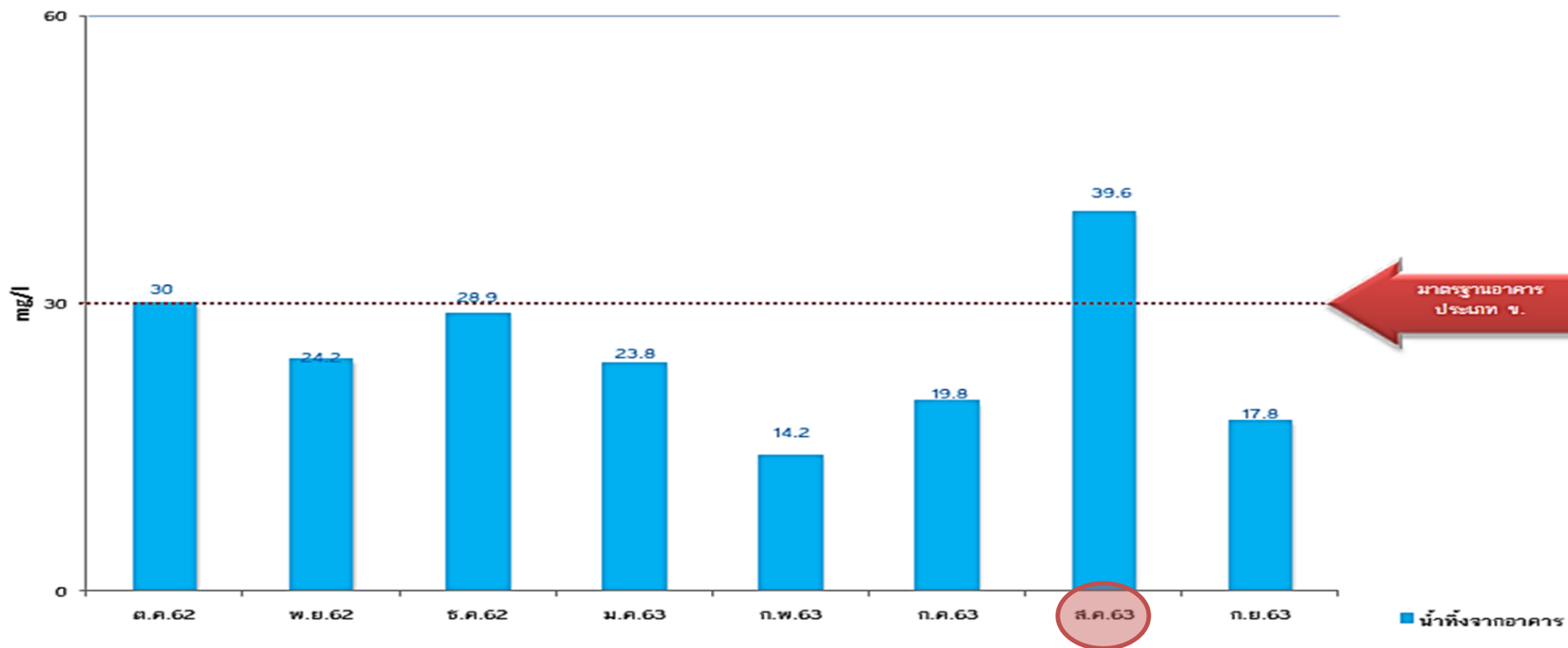
กราฟแสดงค่าบีโอดี (BOD) ของระบบบำบัดน้ำเสียอาคารกรมควบคุมมลพิษ (ระหว่างเดือนตุลาคม 2562 - กันยายน 2563)
