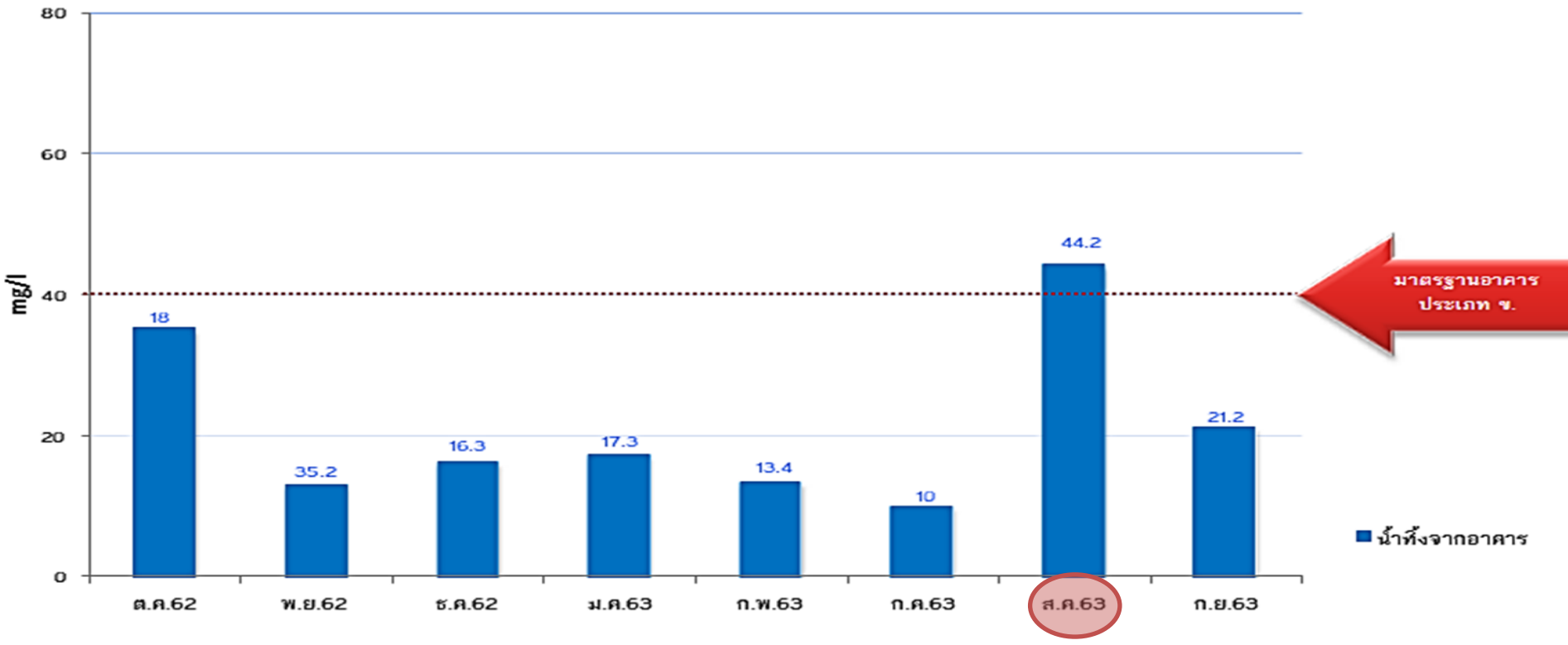
กราฟแสดงค่าของแข็งแขวนลอย (SS) ของระบบบำบัดน้ำเสียอาคารกรมควบคุมมลพิษ (ระหว่างเดือนตุลาคม 2562 - กันยายน 2563)
