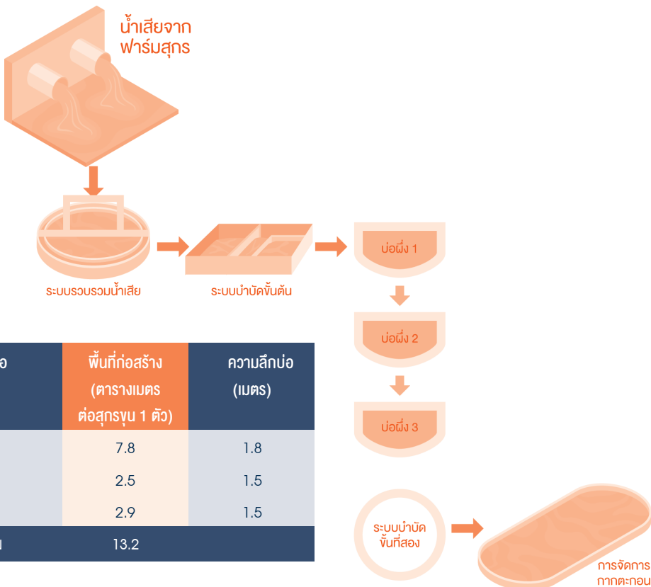
รูปที่ ข - 1 ระบบบ่อผิ้ว
