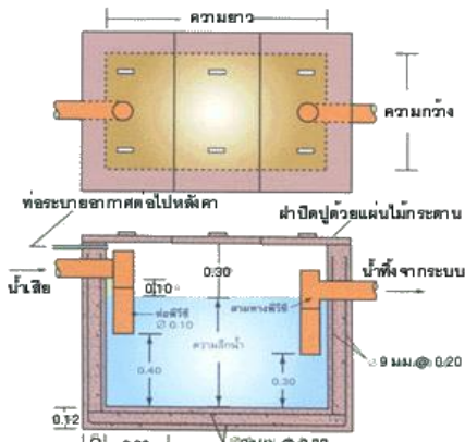
รูปที่ 9 บ่อตกไขมันขนาดใหญ่
