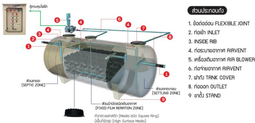
รูปที่ 18 ตัวอย่างถังบำบัดน้ำเสียสำเร็จรูปแบบแอกติเวเตเต็ดสลัดจ์
