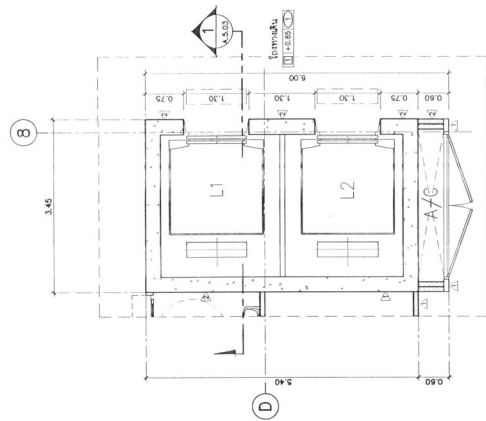
(ชื่องาน) แปลนพื้นที่ 3 มาตราส่วน 1:50
