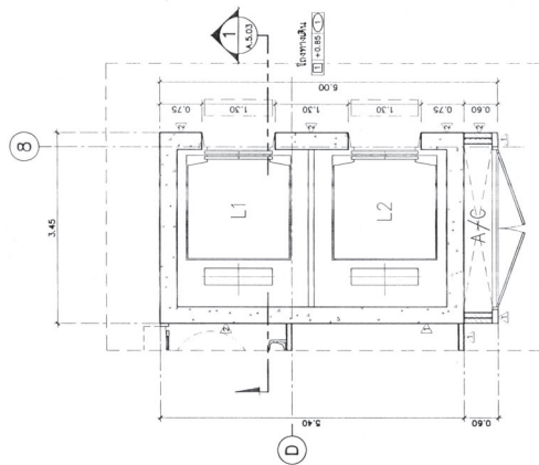
แปลงพันธุ์ชั้นที่ 1 มาตราส่วน 1:50 (ข้อมูลพิมพ์)
