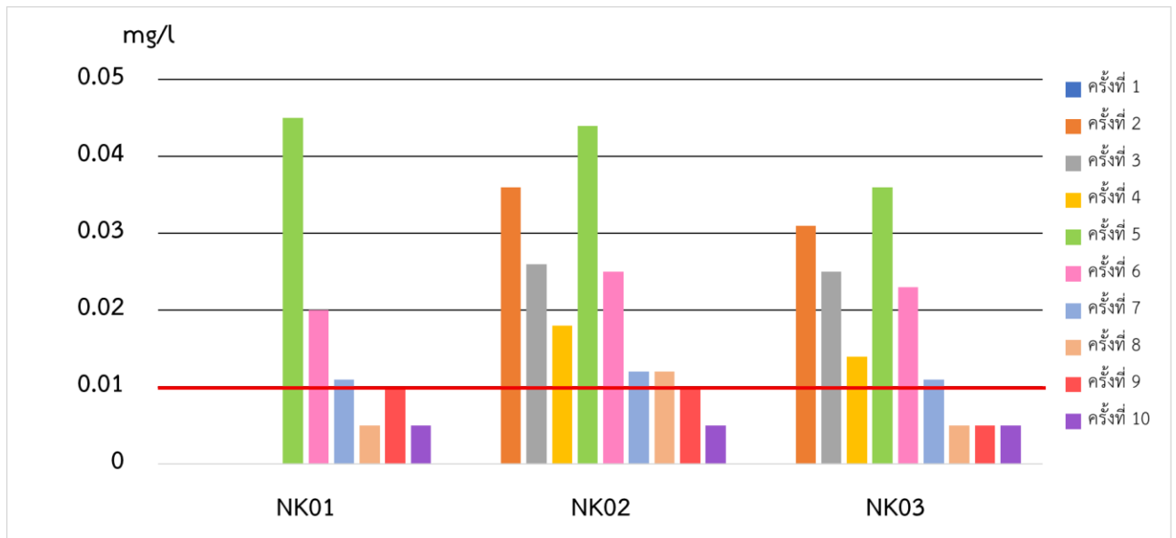
รูปที่ 6 สารหนู (มก./ล.) ในแม่น้ำโขง ระหว่างเดือนมีนาคม – สิงหาคม 2568 และเส้นแสดงระดับสารหนูตามมาตรฐานคุณภาพน้ำในแหล่งน้ำผิวดิน (0.01 มก./ล.) ทั้งนี้ การเก็บตัวอย่างครั้งที่ 1 ไม่มีการตรวจวัดสารหนูในแม่น้ำโขง
