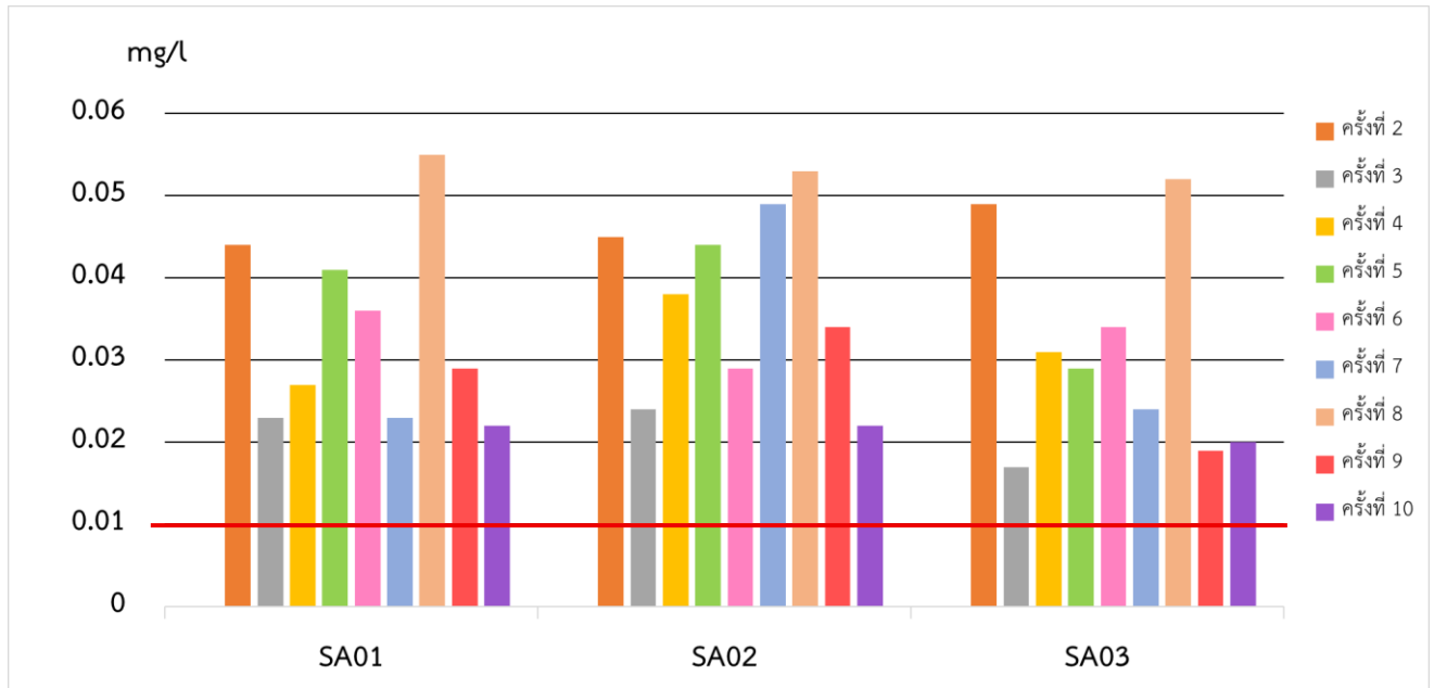
รูปที่ 4 สารหนู (มก./ล.) ในแม่น้ำสาย ระหว่างเดือนมีนาคม – สิงหาคม 2568 และเส้นแสดงระดับสารหนูตามมาตรฐานคุณภาพน้ำในแหล่งน้ำผิวดิน (0.01 มก./ล.) ทั้งนี้การเก็บตัวอย่างครั้งที่ 1 ไม่มีการตรวจวัดสารหนูในแม่น้ำสาย
