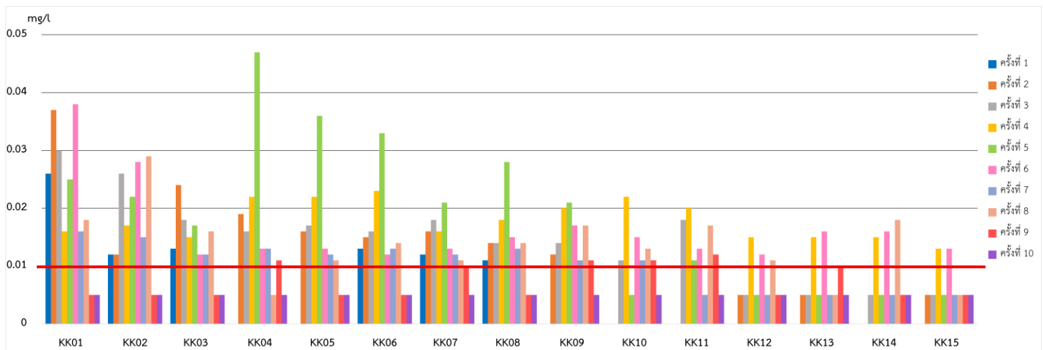
รูปที่ 3 สารหนู (มก./ล.) ในแม่น้ำกก ระหว่างเดือนมีนาคม - สิงหาคม 2568 และเส้นแสดงระดับสารหนูตามมาตรฐานคุณภาพน้ำในแหล่งน้ำผิวดิน ( 0.01 มิลลิกรัมต่อลิตร หรือ มก./ล.)
