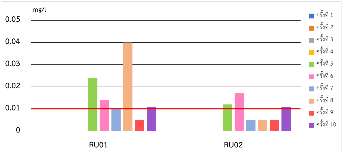
รูปที่ 5 สารหนู (มก./ล.) ในแม่น้ำรวก ในเดือนมิถุนายน เดือนกรกฎาคม และสิงหาคม และเส้นแสดงระดับสารหนูตามมาตรฐานคุณภาพน้ำในแหล่งน้ำผิวดิน (0.01 มก./ล.)
