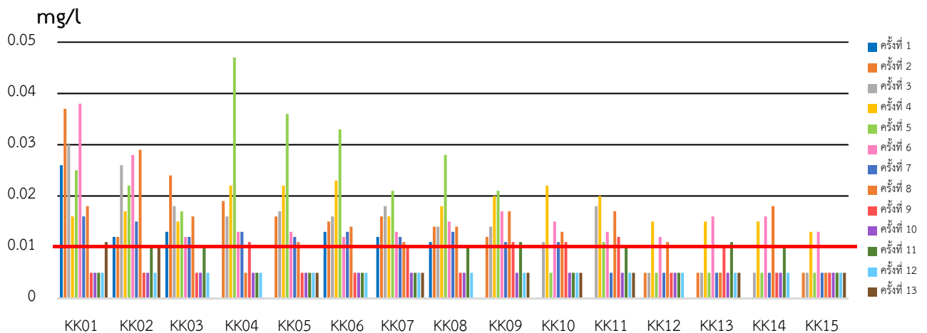
รูปที่ 3 สารหนู (มก./ล.) ในแม่น้ำกก ระหว่างเดือนมีนาคม – พฤศจิกายน 2568 และเส้นแสดงระดับสารหนูตามมาตรฐานคุณภาพน้ำในแหล่งน้ำผิวดิน (0.01 มิลลิกรัมต่อลิตร หรือ มก./ล.)
