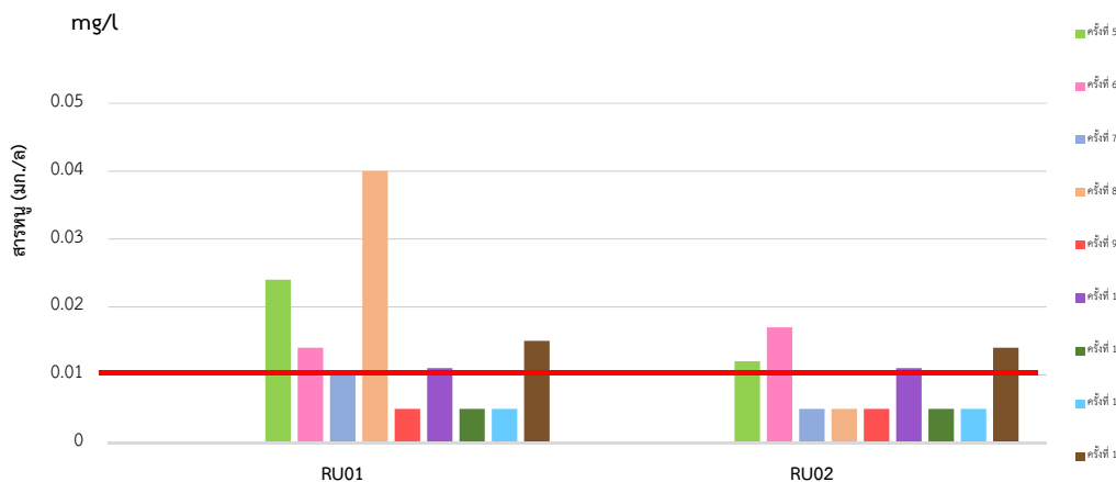
รูปที่ 5 สารหนู (มก./ล.) ในแม่น้ำรวก ในเดือนมิถุนายน – พฤศจิกายน 2568 และเส้นแสดงระดับสารหนูตามมาตรฐานคุณภาพน้ำในแหล่งน้ำผิวดิน (0.01 มก./ล.)
