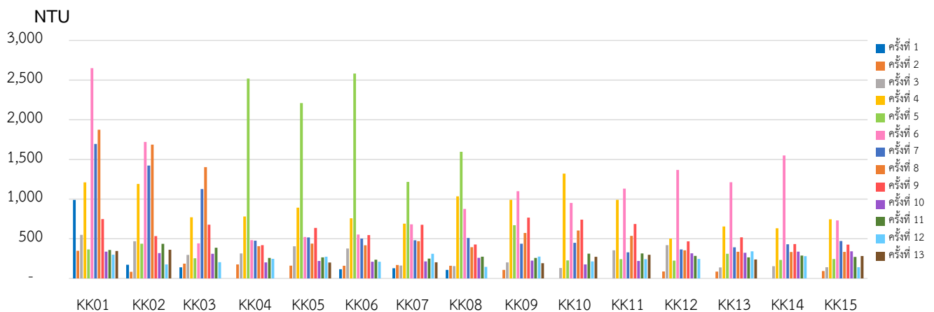
รูปที่ 2 ความขุ่นในแม่น้ำกก ระหว่างเดือนมีนาคม – พฤศจิกายน 2568
